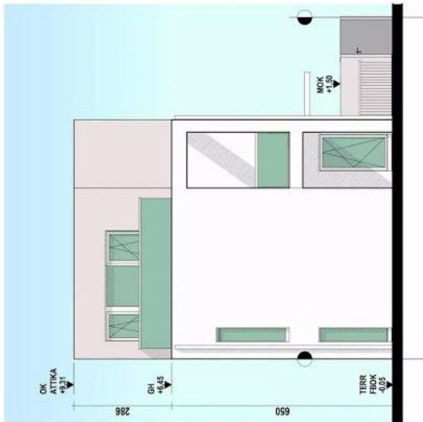
ANSICHT WEST HAUS 2
